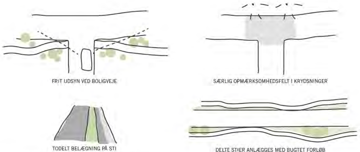
FIG. 39: PRINCIPPER FOR UDFORMNING AF PERIMETERVEJ
